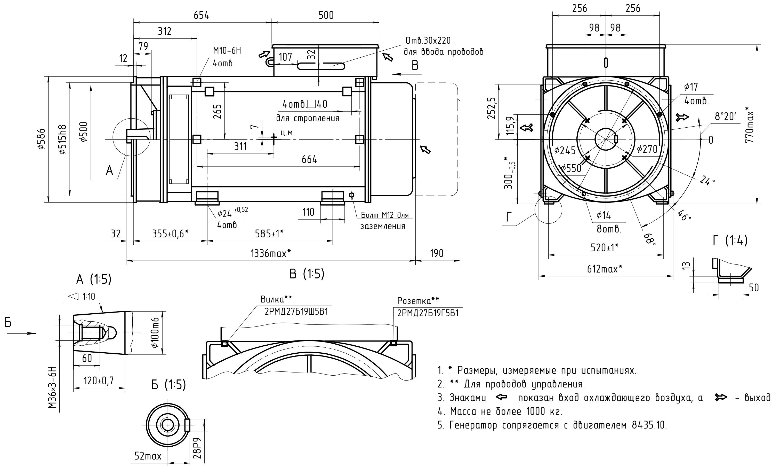
Рисунок 15 - Габаритный чертеж генератора мощностью 250 кВт
